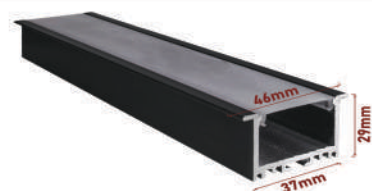
توکار سایز: 29*37 میلی متر
