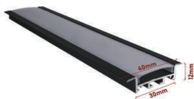
توکار سایز: 30*12 میلی متر
