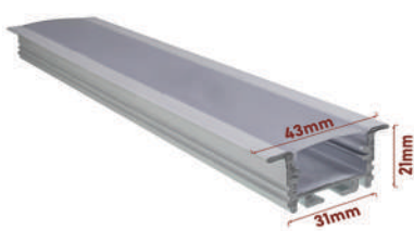
توکار سایز: 31*21 میلی متر
